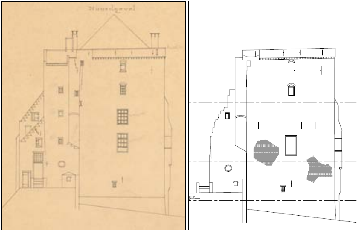
De noordgevel van kasteel De Nijenbeek, volgens opmetingen van Adolph Mulder (links, 1884) en Braaksma & Roos architectenbureau (rechts, 2010).
