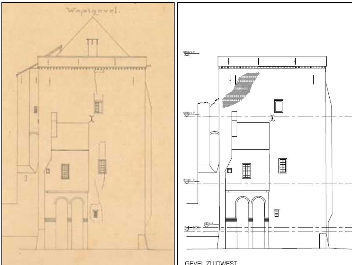
De westgevel van kasteel De Nijenbeek, volgens opmetingen van Adolph Mulder (links, 1884) en Braaksma & Roos architectenbureau (rechts, 2010).
