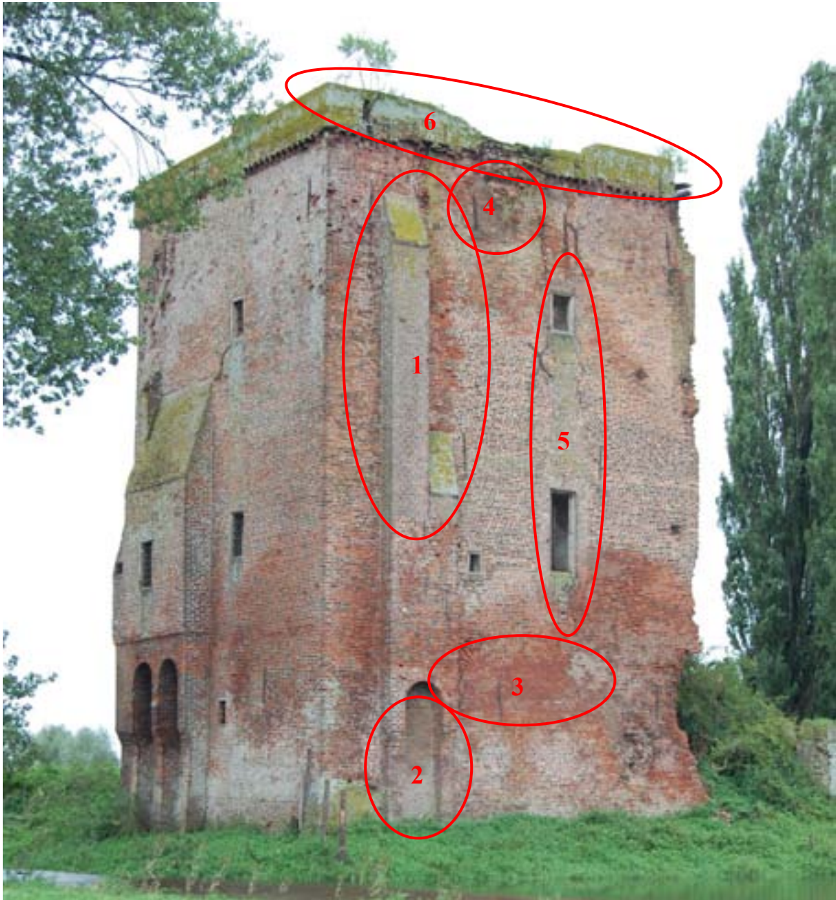
Overhoeks aanzicht van de zuidgevel. Met de rode ovalen zijn de voornaamste wijzigingen na de Middeleeuwen aangegeven. Het privaat is in de 17 de eeuw verhoogd (1), waarbij ook pilasters aan de onderzijde zijn toegevoegd (2). Bij 3 is een herstelling uit de 18 de of 19 de eeuw te zien, vermoedelijk ter plaatse van een dichtgezet kelderlicht. Ook 4 is een herstelling. Bij 5 zijn de laat-19 de -eeuwse aanpassingen van de vensters te herkennen. De muurkroon is vernieuwd in de late 18 de eeuw of vroege 19 de eeuw (6).
