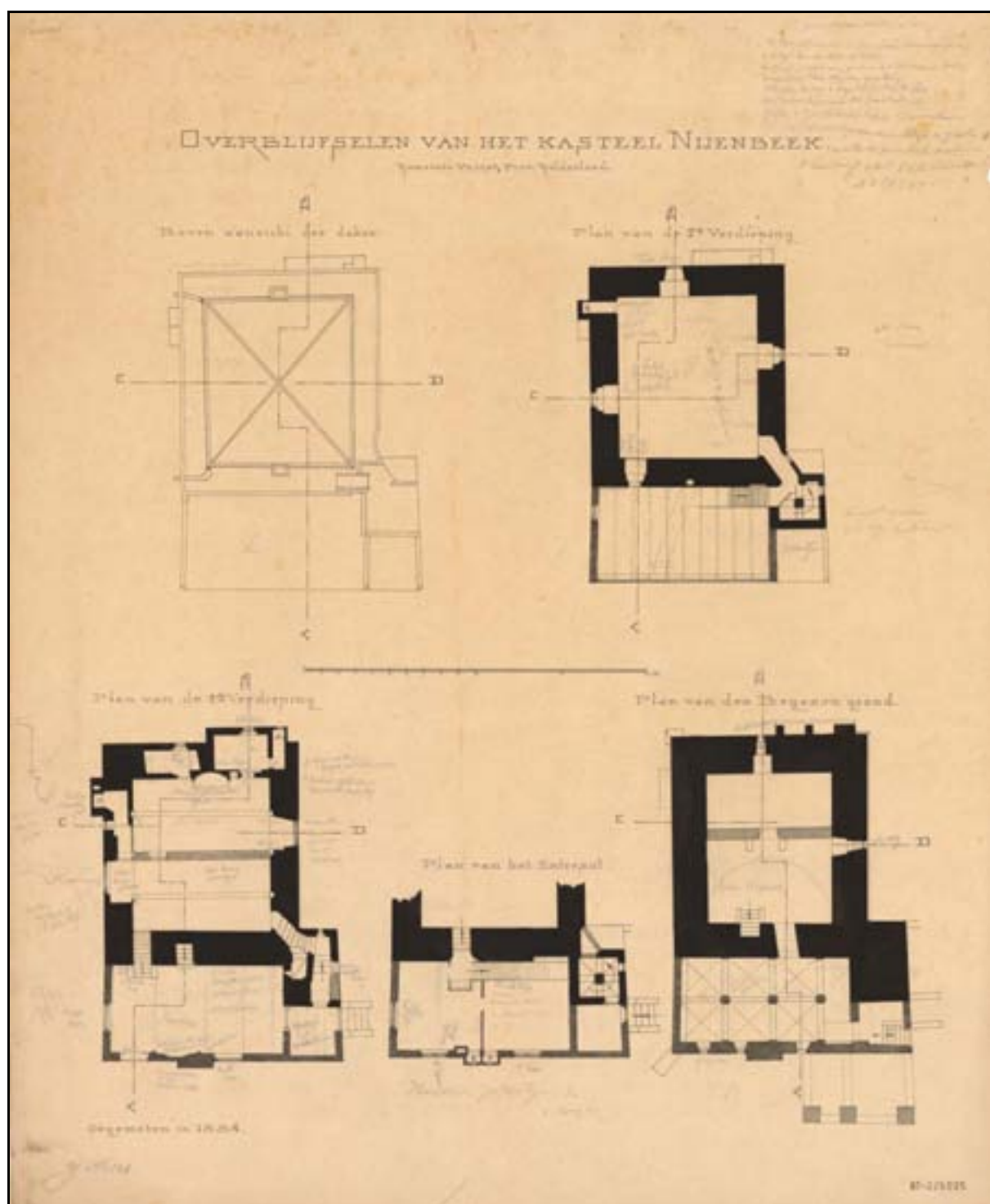
Plattegronden van het kasteel De Nijenbeek, naar een opmeting en tekening door A. Mulder uit 1884 (collectie Rijksdienst voor het Cultureel Erfgoed).
