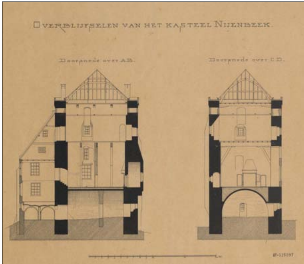
Doorsneden van het kasteel De Nijenbeek, naar een opmeting en tekening door A. Mulder uit 1884 (collectie Rijksdienst voor het Cultureel Erfgoed).
