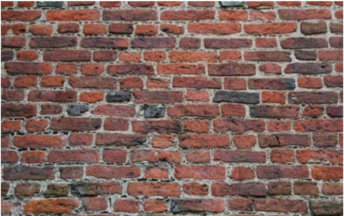
Detail van het metselwerk aan de voet van de noordgevel, gemetseld in Vlaams verband.
