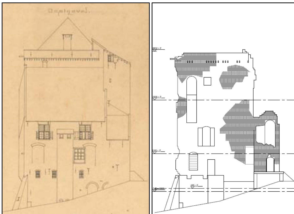
De oostgevel van kasteel De Nijenbeek, volgens opmetingen van Adolph Mulder (links, 1884) en Braaksma & Roos architectenbureau (rechts, 2010). Op de opmetingstekening van Mulder valt de aanbouw tegen de oostgevel nog te herkennen.
